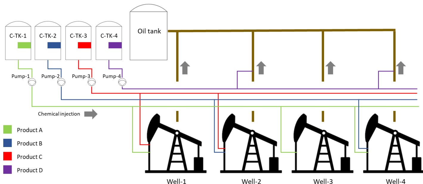
Figura 1 – Diagrama de injeção química: Site 1 (Genérico)
